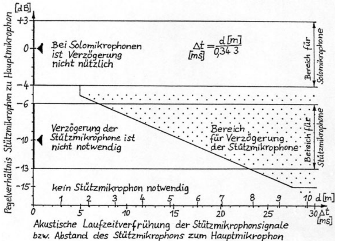
Grenzwertfestlegung für die Signalverzögerung der Stütz- und Hauptmikrofon signale als Funktion des Pegelverhältnisses und des Abstands
