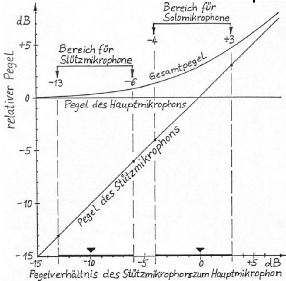
Leistungssumme von Haupt- und Stütz- und Hauptmikrofon als Funktion des relativen Pegels
