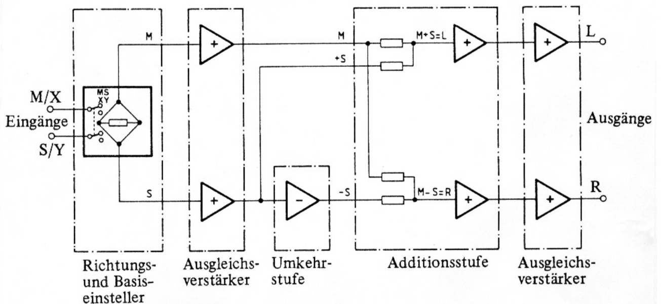
Schaltbild des Richtungsmischers
